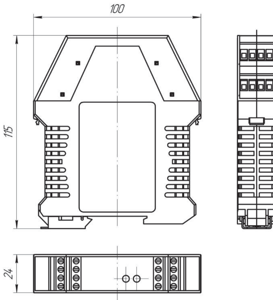
Рисунок А.1 – Габаритные размеры Источника (не более), мм.
