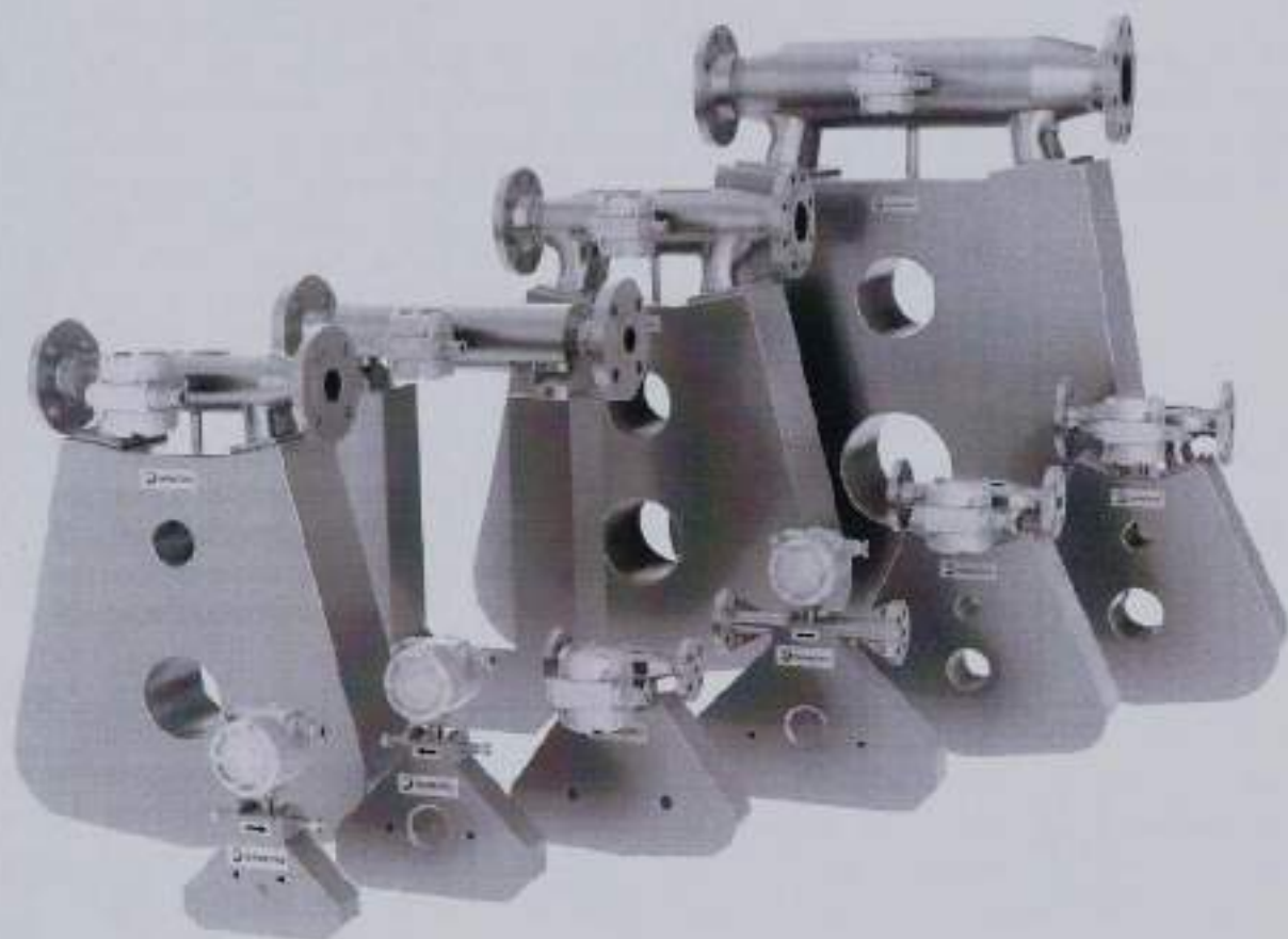
Рисунок 1 - Датчики расходомера
