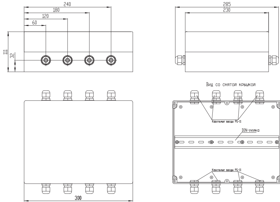
Рисунок А.2 Соединительная коробка IP 65, корпус из ABS-пластика (опция – box1) Примечание: Размеры «для справок»
