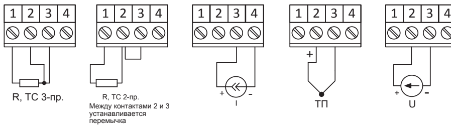
Рисунок 1.3 Подключение датчиков к каналам АВ.
