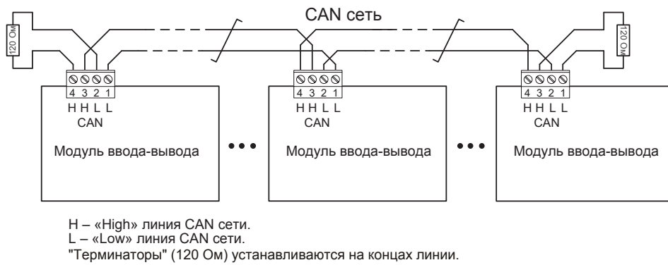
Рисунок Б.1 Подключение модулей в сеть по CAN-интерфейсу
