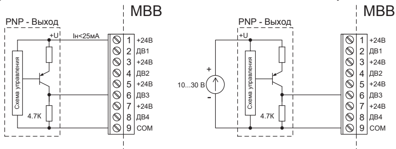
Рисунок 1.9 Подключение датчиков с PNP-выходом.
