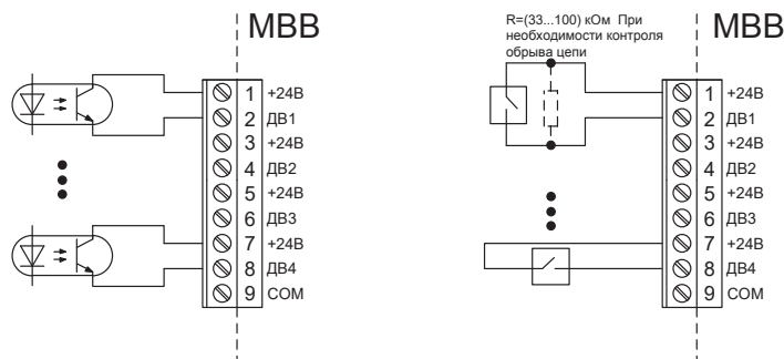
Рисунок 1.8 Подключение датчиков с выходным сигналом типа "сухой" контакт.
